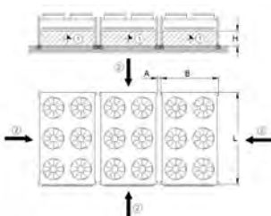
Ustawienie w zestawie
