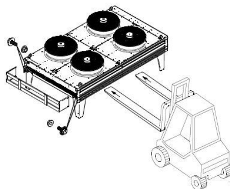
Rozpakowanie urządzeń o konstrukcji poziomej
